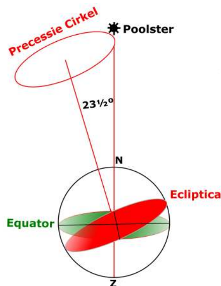
Precessie van de aardas
