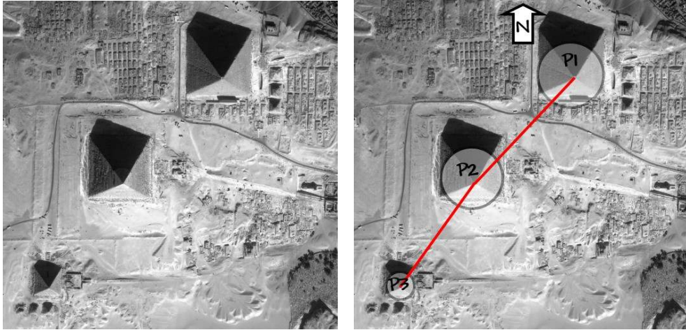
Luchtfoto van het plateau van Gizeh, rechts de posities van de planeten
