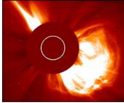
Zonnevlammen op 4 november 2003 (NASA)
