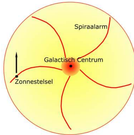
Bovenaanzicht van de spiraalarmen van de Melkweg
